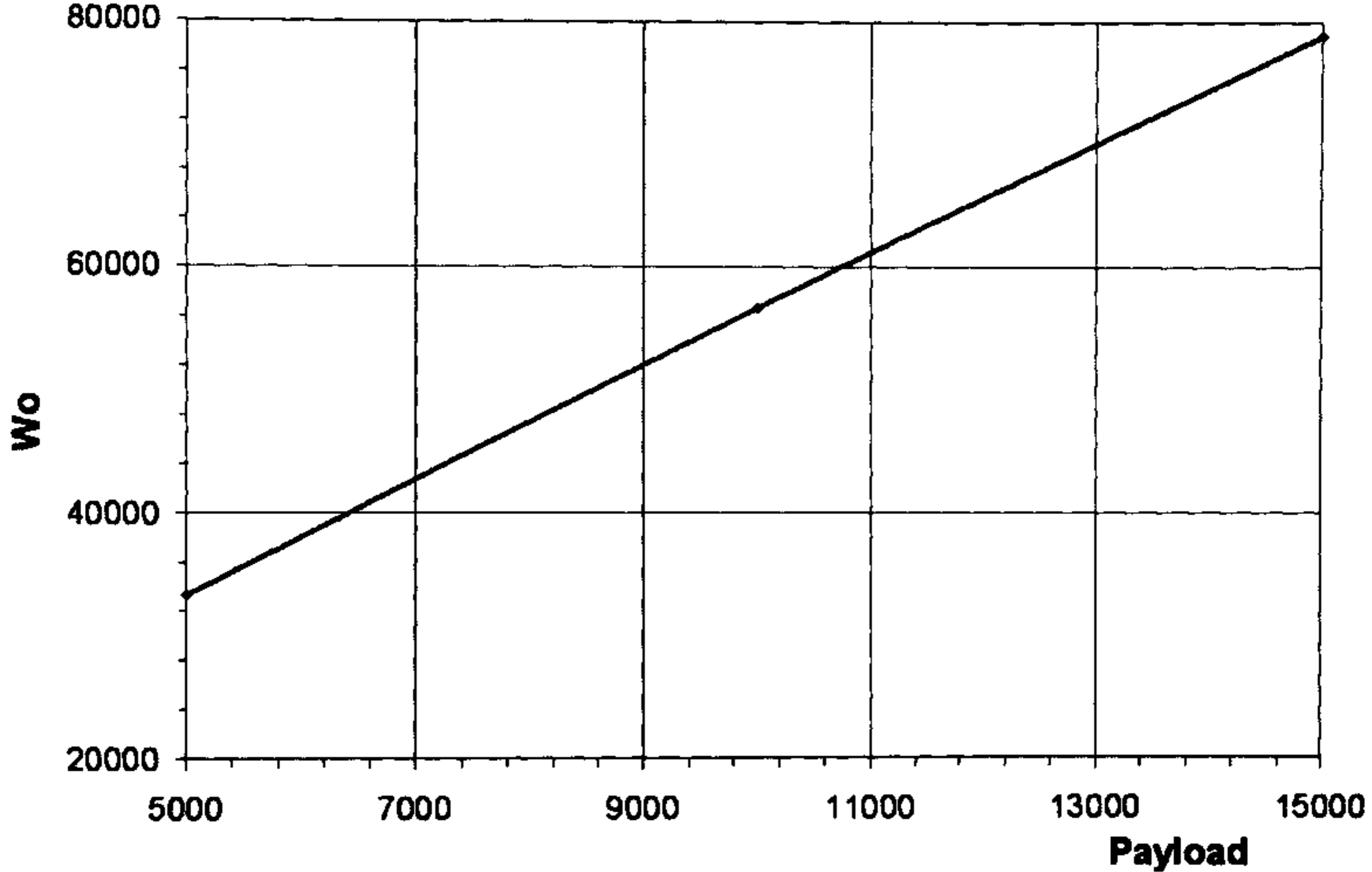
Fig. 3.13 Payload trade.
