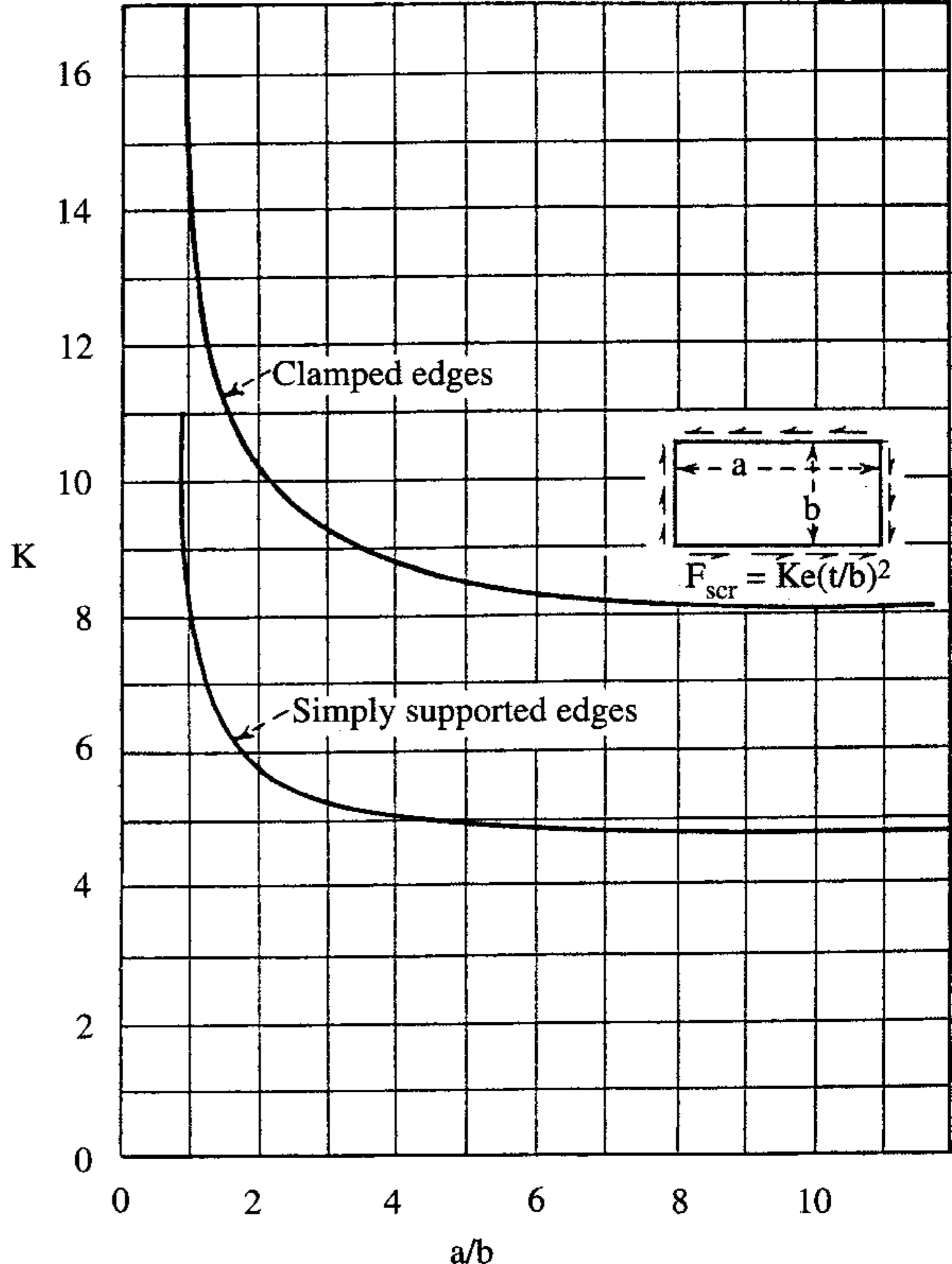
Fig. 14.42 Shear web buckling (NACA TN3781).
